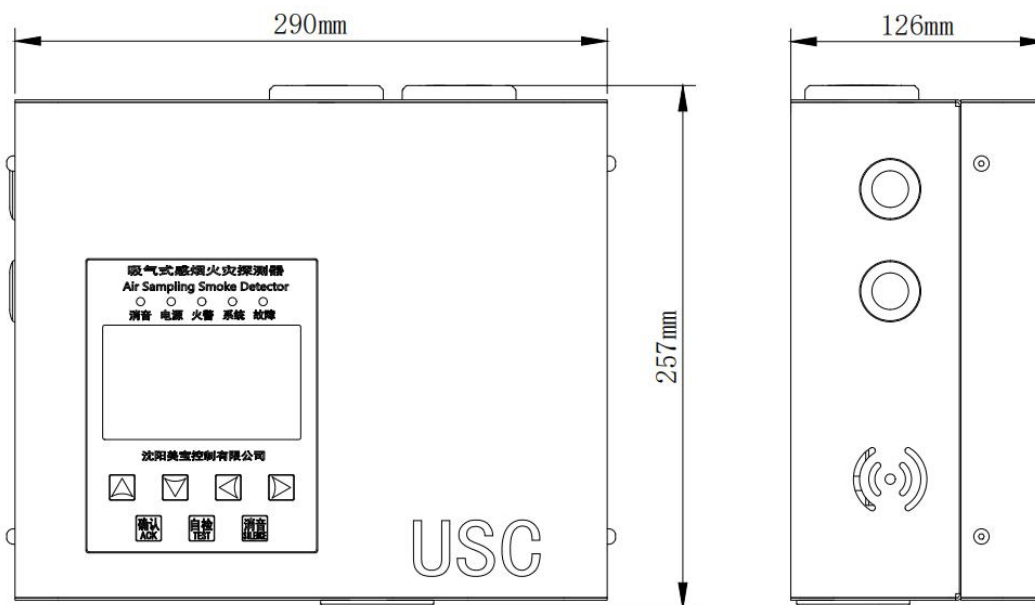
USC4922 吸气式感烟火灾探测器尺寸图 (5-1)
