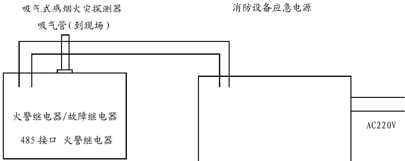
系统接线图 (3-3-1)
