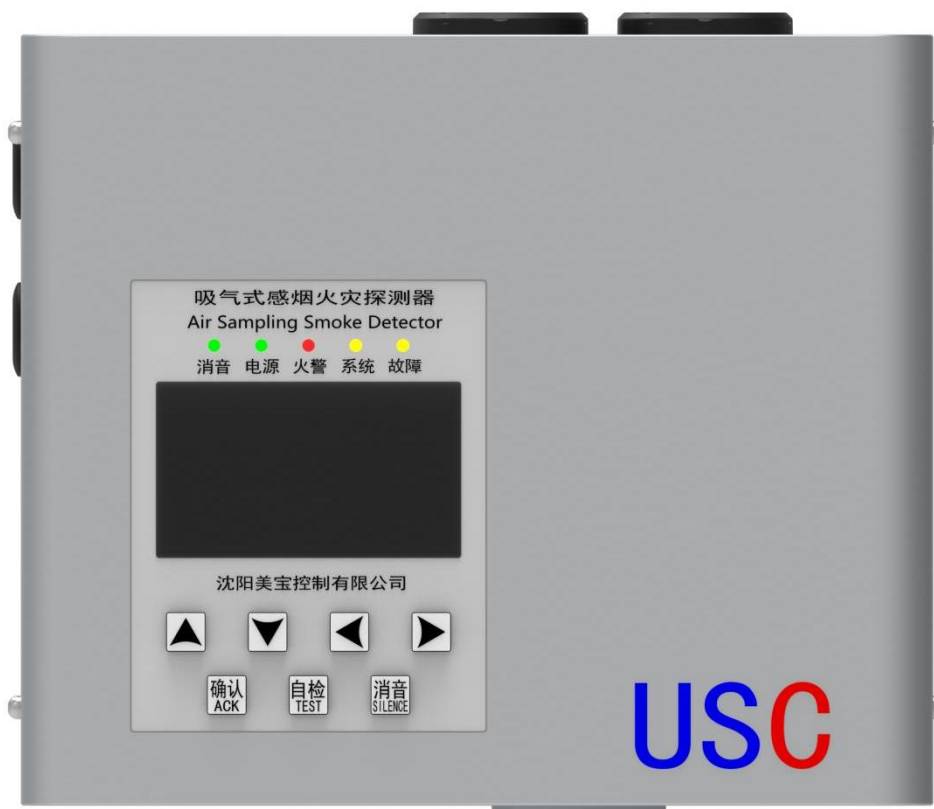
USC4922 吸气式感烟火灾探测器整机图（3-1-1）
