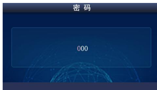
密码界面 (7-2-14)
